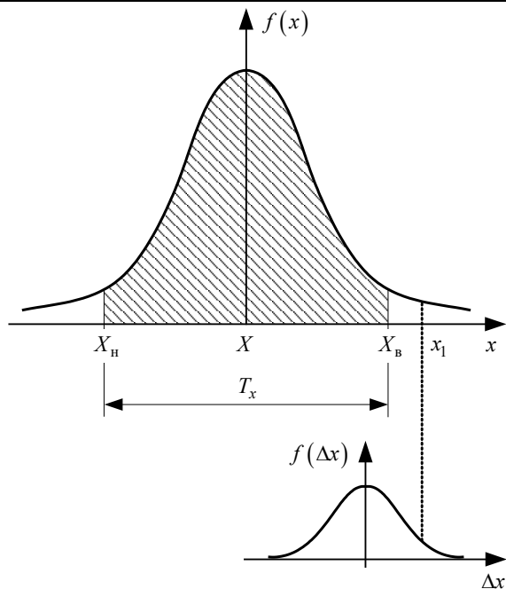
Рис. 2.53. Формирование распределения плотности вероятности f(x) ошибок контроля
