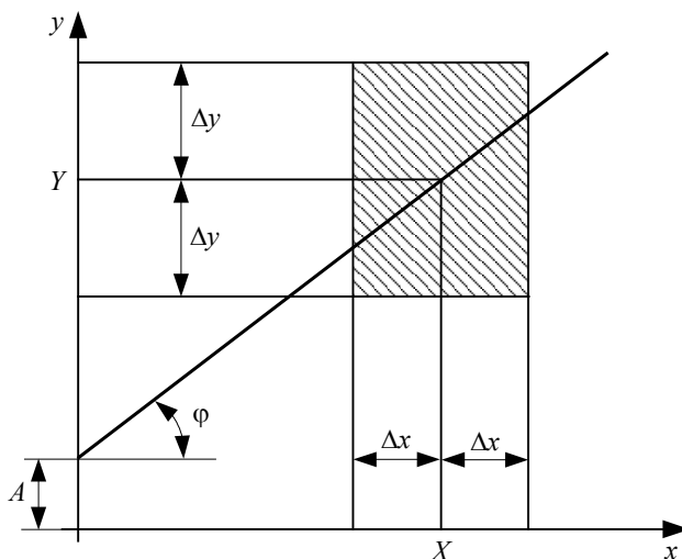
Рис. 2.51. Аппроксимация линейной функциональной зависимости
