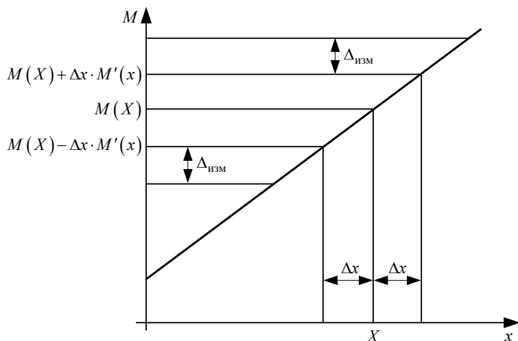
Рис. 2.52. Формирование погрешности испытания
