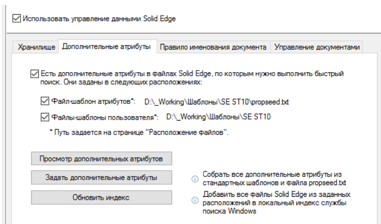
Рис. 2.42. Дополнительные атрибуты
