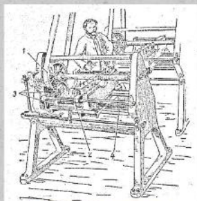
Токарный станок, изготовленный на Тульском оружейном заводе в середине 18 века
