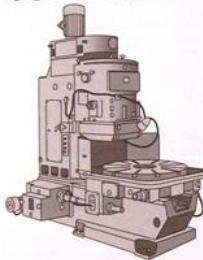
Гравировальный копировально-фрезерный станок с пантографом
