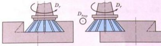
Паза типа «ласточкин хвост»
