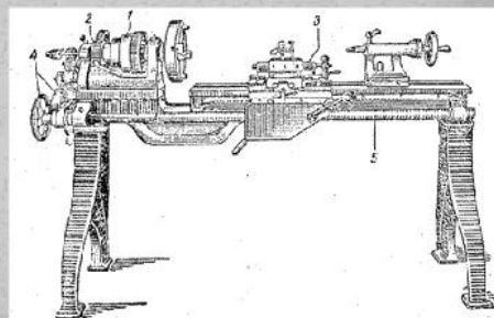
Токарный станок середины 19 века со ступенчатым шкивом
