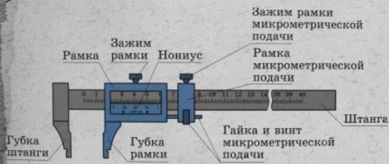
Штангенциркуль ШЦ-III
