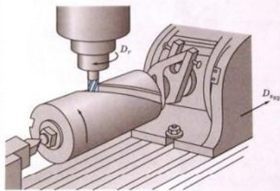
Винтовых поверхностей Пальцевой фрезой
