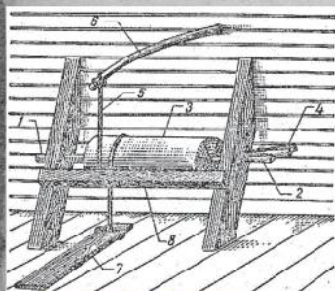
Старинный русский токарный станок
