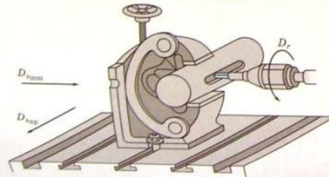
Шпоночной канавки
