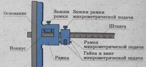
Штангенглубиномер
