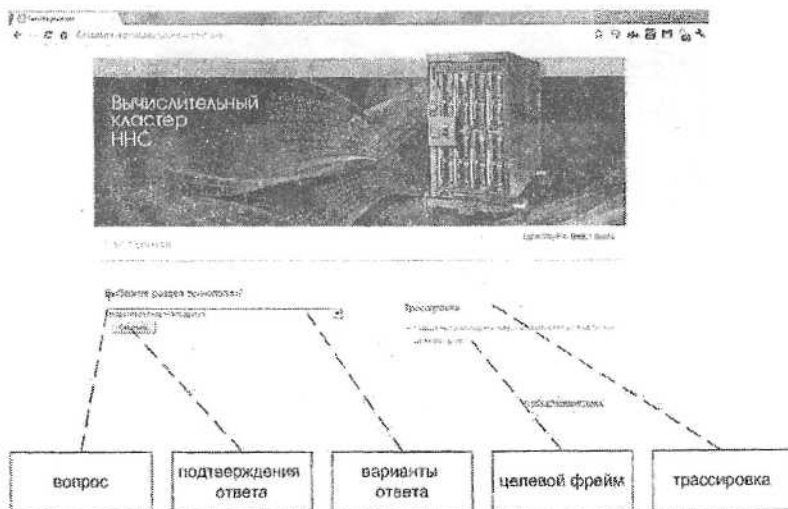
Рисунок 4.4 - Декомпозиция объектов
