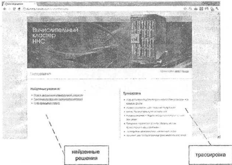
Рисунок 4.7 - Найденные решения
