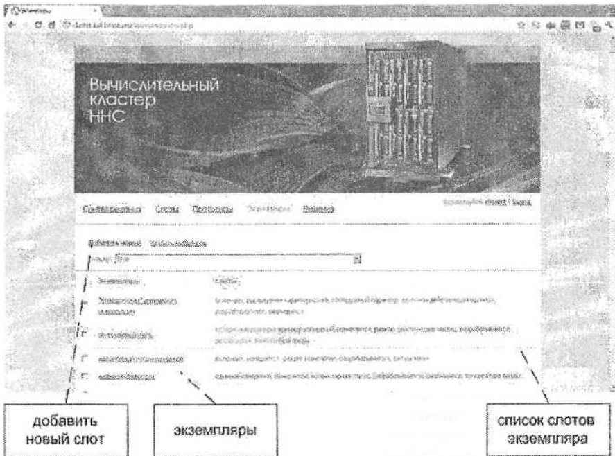
Рисунок 5.6 - Модуль экземпляры
