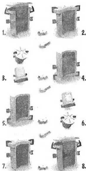
Рисунок 7.3 - «Покадровое» представление процесса получения оболочковых полуформ: 1 - установка крышки бункера с закрепленной на ней и нагретой стальной полумоделью на бункер; 2 - закрепление крышки на бункере; 3,4- первая стадия: поворот бункера в нижнее рабочее положение (формовочная смесь, состоящая из песка и терморезактивной смолы,
