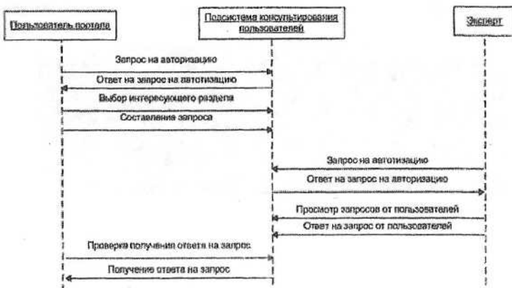
Рисунок 5.10 - Сценарий использования подсистемы консультирования пользователей
