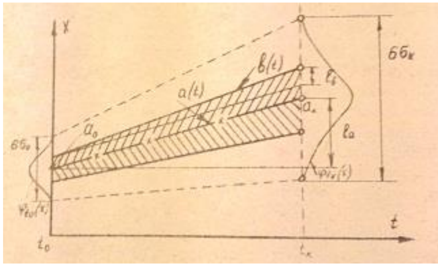
Рис. 6. Точностная диаграмма технологического процесса: a(t) - линия изменения среднего значения параметра качества; b(t) - линия изменения среднего квадратического отклонения; f_{L_0}(x) f_{L_x}(x) - мгновенные распределения; a_0, a_x - центр группирования погрешностей в мгновенных распределениях, t_0 t_x - начальное и конечное значения элемента, ----- границы изменения полей расстояния погрешностей.
