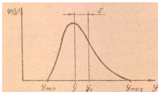
Рис. I. Распределение производственных погрешностей параметра
