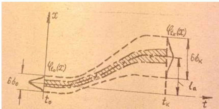
Рис. 13. Точностная диаграмма технологического процесса при нелинейных функциях a(t) и b(t) с точками перегиба
