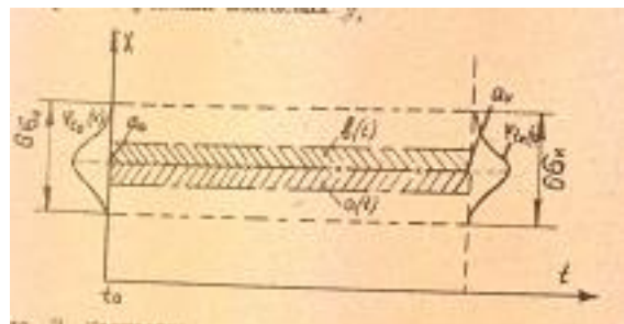
Рис.7. Точностная диаграмма технологического процесса при гауссовском законе полного распределения погрешностей.
