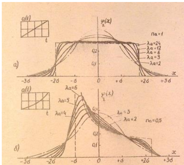
Рис. 8. Полные распределения погрешностей параметра качества изделий при различных функциях a(t) : \lambda_a - показатель степени функции a(t) ; _____ - _____ гауссовское распределение, - - - - - предельный закон распределения.
