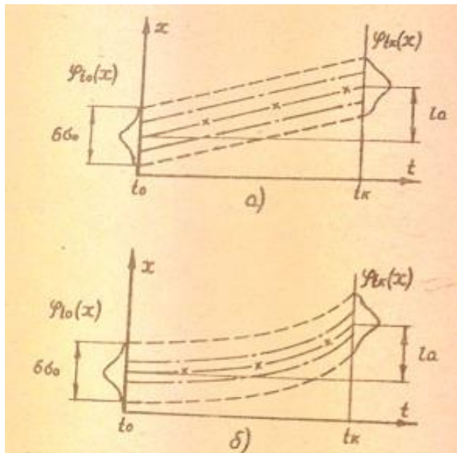
Рис. 9. Точностные диаграммы технологических процессов при линейной (а) и ускоренно возрастающей (б) функции a(t)
