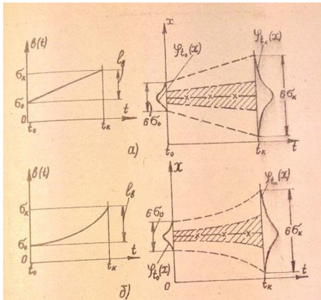
Рис. 11. Точностные диаграммы технологических процессов при различных функциях b(t) .
