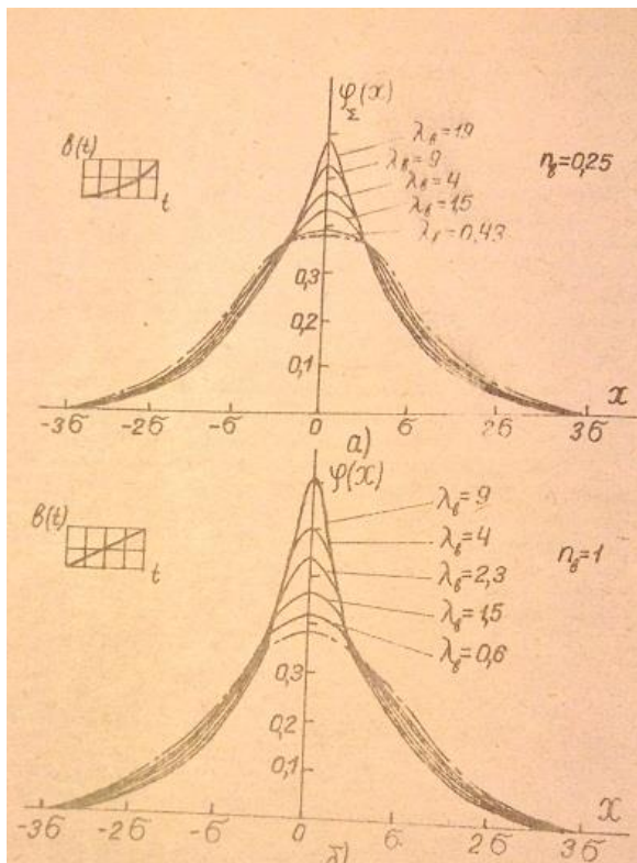
Рис. 10. Полные распределения при различных функциях \sigma(t) ; n_g - показатель степени функции \sigma(t) ; _____ - гауссовское распределение
