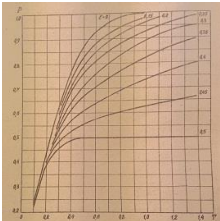
Рис. 4. Вероятность выхода годных изделий при гауссовском законе распределения погрешностей параметра качества
