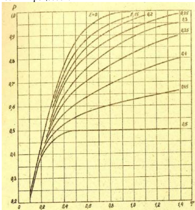
Рис. 4. Вероятность выхода годных изделий при гауссовском законе распределения погрешностей параметра качества
