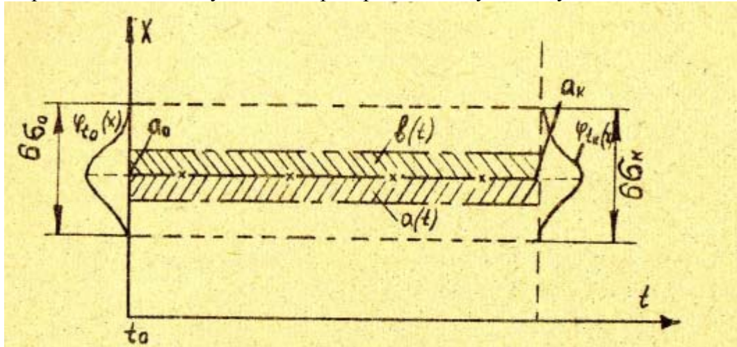
Рис. 7. Точностная диаграмма технологического процесса при гауссовском законе полного распределения погрешностей
