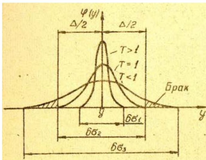
Рис. 2. Гауссовские распределения при различных коэффициентах точности T
