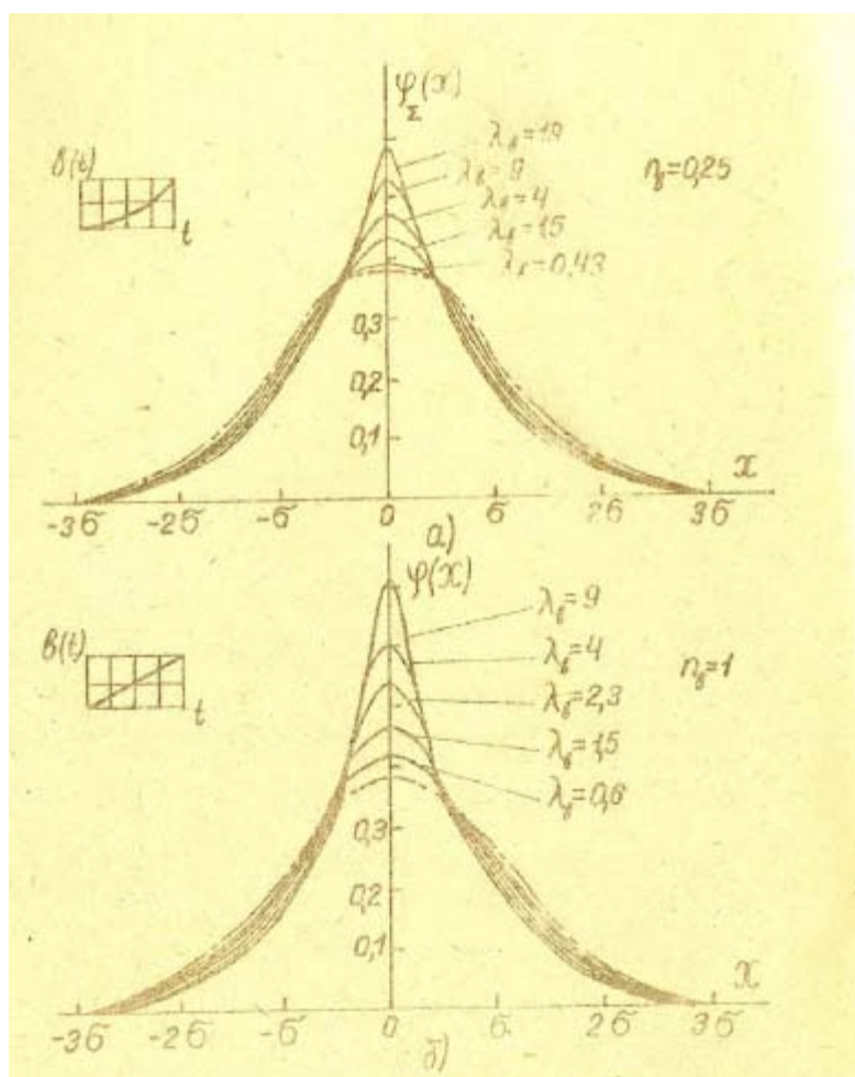
Рис. 10. Полные распределения при различных функциях b(t) : n_b – показатель степени функции b(t) ; ..... - гауссовское распределение
