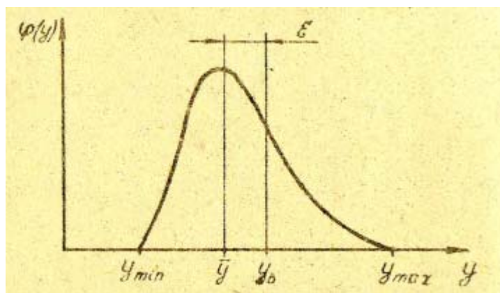
Рис. 1. Распределение производственных погрешностей параметра качества изделия
