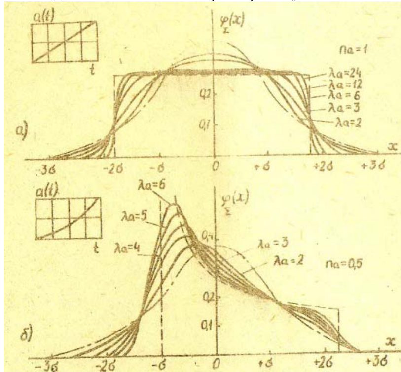
Рис. 8. Полные распределений погрешностей параметра качества изделий при различных функциях a(t) ; n_a - показатель степени функции a(t) ; ..... гауссовское распределение; ..... предельный закон распределения
