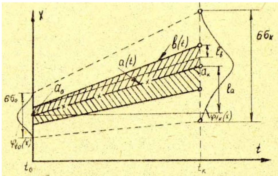
Рис. 6. Точностная диаграмм технологическою процесса: a(t) - линия изменения среднего значения параметра качества; b(t) линия изменения среднего квадратического отклонения; \varphi_{t_0}(x) , \varphi_{t_k}(x) мгновенные распределения; a_0 , a_k - центры группирования погрешностей в мгновенных распределениях; t_0 , t_k - начальное и конечное значения аргумента; ----- - границы изменения полей рассеяния погрешностей
