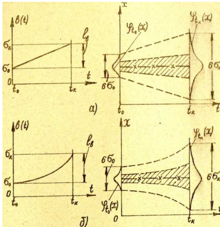
Рис. 11. Точностные диаграммы технологических процессов при различных функциях b(t)
