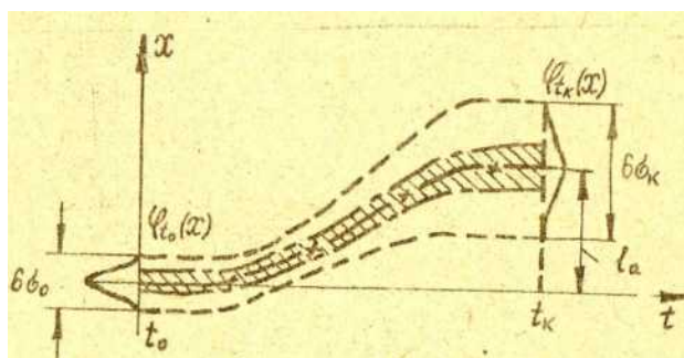
Рис. 13. Точностная диаграмма технологического процесса при нелинейных функциях a(t) и b(t) с точками перегиба
