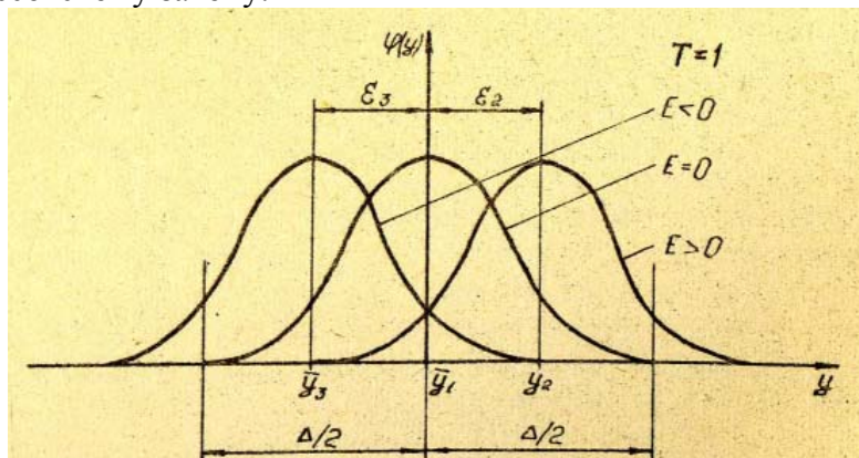
Рис. 3. Гауссовские распределения при различных коэффициентах смещения \varepsilon
