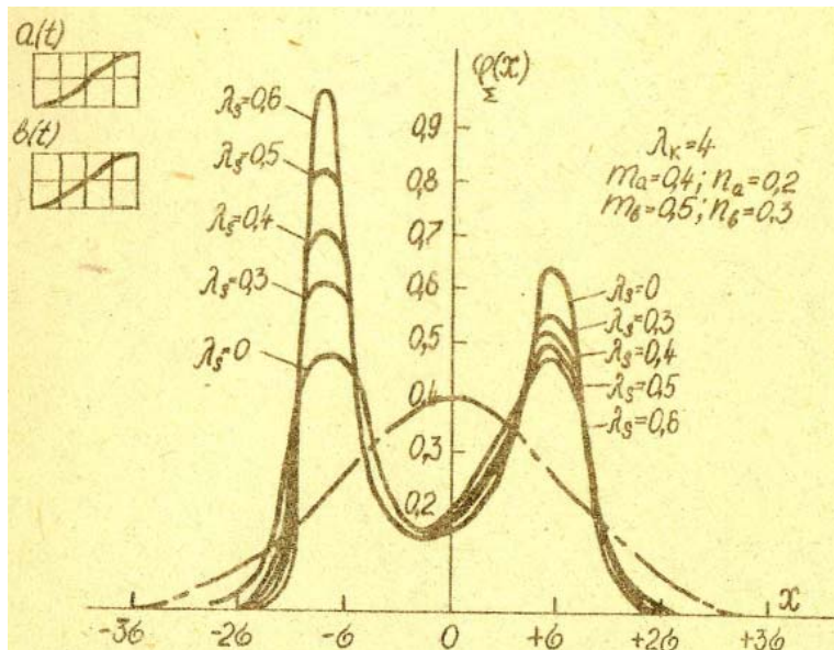
Рис. 12. Дачные распределения при нелинейных функциях a(t) и b(t) с точками перегиба: ..... - гауссовское распределение; n_a и n_b - показатели степени функций a(t) и b(t) соответственно; m_a и m_b - абсциссы точек перегиба в функциях a(t) и b(t) соответственно
