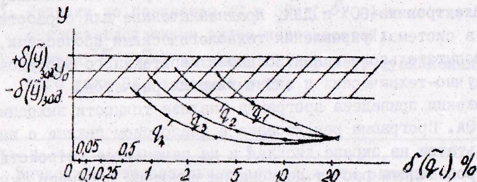
Рис. 2. Семейство графиков \delta(\bar{y})_{расч.элем} = f[\delta(\bar{q}_i)] для комплектующих ИС и ЭРЭ
