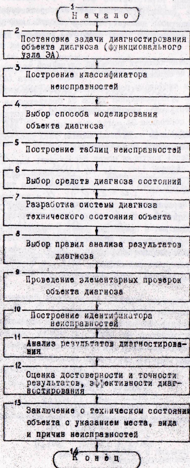
Рис. 4. Обобщенный алгоритм технического диагностирования функциональных узлов ЭА
