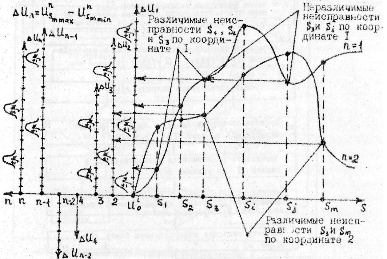
Рис. 7. Анализ различимости неисправностей
