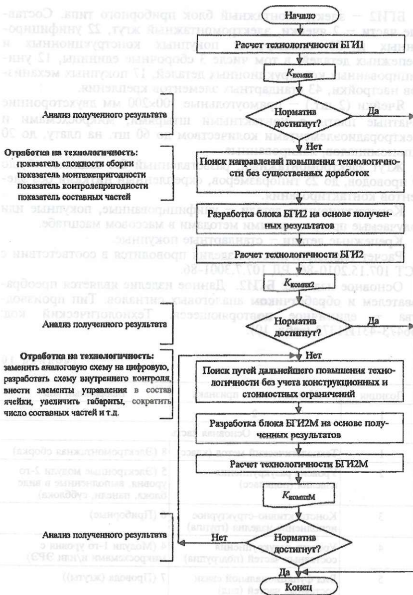
Рис. 3. Схема алгоритма отработки изделия БГИ1 на технологичность
