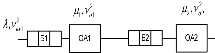
Рис. 4.3 Двухфазная сеть массового обслуживания
