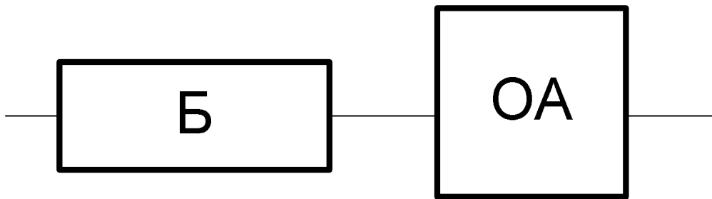
Рис. 3.6 СМО типа M/\underline{E_k}/1
