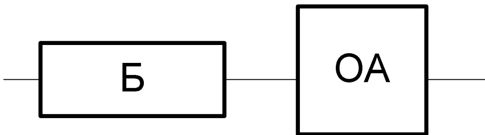
Рис. 3.5 СМО типа M/ E k /1
