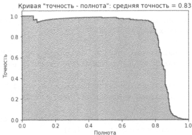
Рис. 2.8. Кривая “точность — полнота” градиентного бустинга XGBoost
