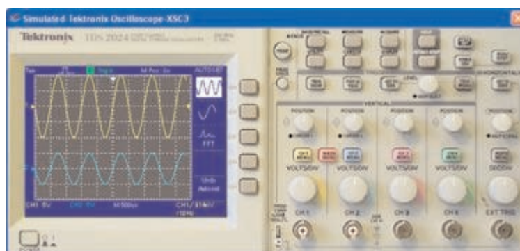
Рисунок 40 – Лицевая панель осциллографа Tektronix
