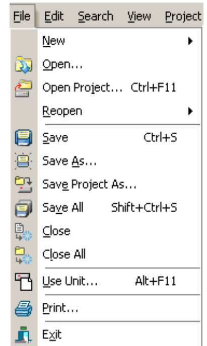
Рисунок 2 – Пункт File
