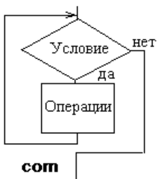
Рисунок 2 – Цикл-пока
