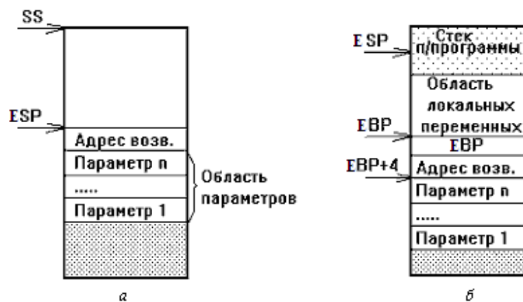
Рисунок 4 – Содержимое стека:
